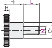
带台阶 外螺纹型 HAU96/97/98/99
