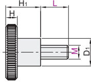
带台阶 外螺纹型 HAU95
