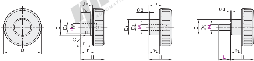
销钉固定型 HAV51
