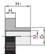
内螺纹型 HAW38/39
