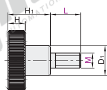
带台阶 外螺纹型 HAW36/37
