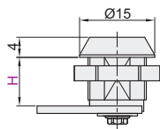
子弹形锁芯 XAS03
