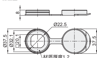
防尘盖
