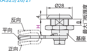
三角形 XAS05/06/07 正方形 XAS15/16/17 双牙形 XAS25/26/27
