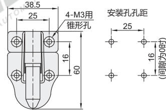
无锁型·碟型 HGA42
