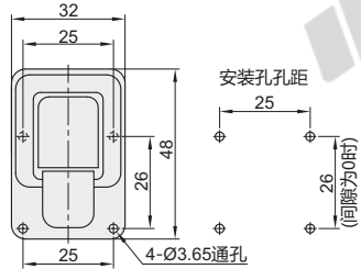
无锁型·方型 HGA41
