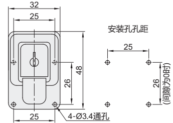
带锁型·方型 HGA46
