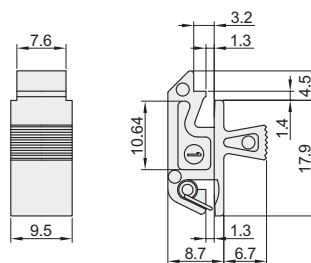
防震动型 HGA23
