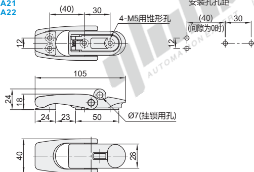
防尘型 HGA21 HGA22
