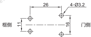
安装孔孔距
