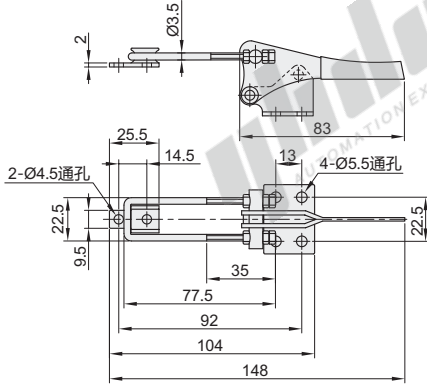
中载型 HGA66
