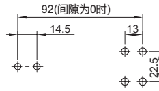
安装孔间距
