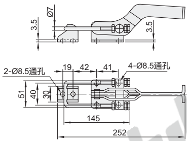
安装孔间距
