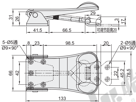
重载型 HGA60
