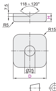
重载型·方形 WAJ73
