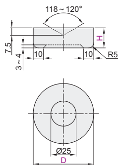
中轻载型·圆形 WAJ71
