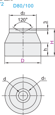
重载型·圆形 WAJ72
