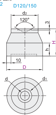
重载型·圆形 WAJ72
