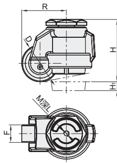
螺杆活动型 CXB01
