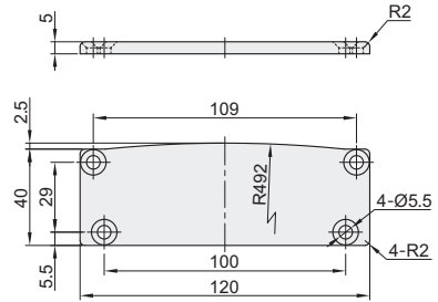
AGT50-A-40120
