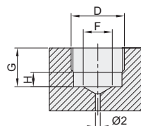
底座尺寸图
